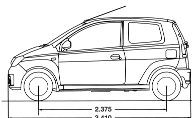
CUORE 3-Türer (Angaben in mm)
