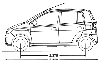
CUORE 5-Türer (Angaben in mm)
