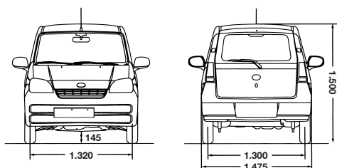
CUORE 3-Türer/5 Türer (Angaben in mm)
